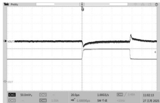
图 8. 1.5V 输出瞬态响应
