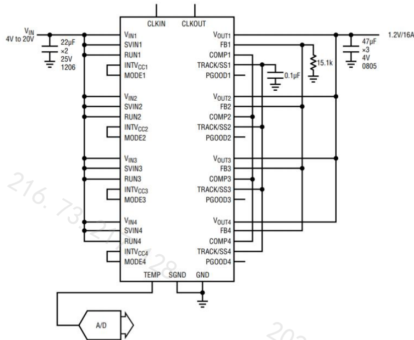
图 22. 具有温度监控功能的 4V 至 20V 输入、4 相、1.2V、16A 设计
