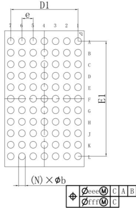
底视图
