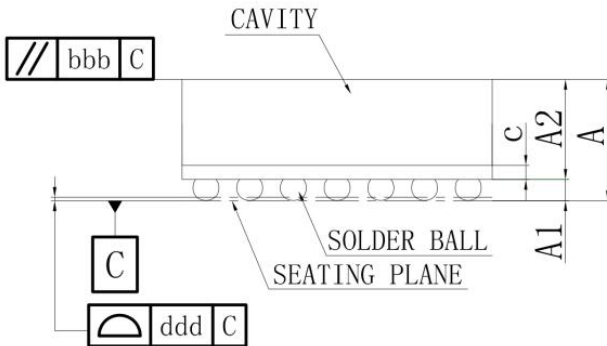
侧视图
