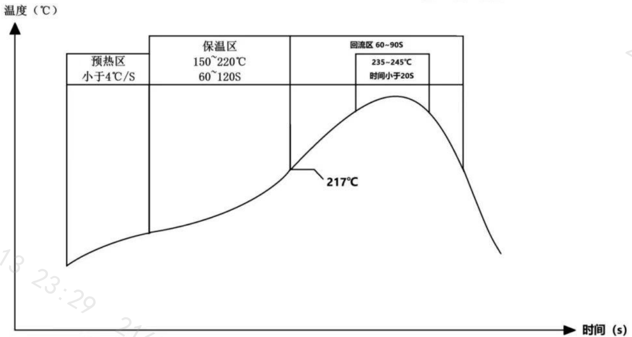
图 25. GC4644N 回流焊温度曲线图
