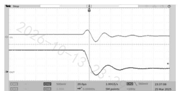
图 15. 3A 负载短路
