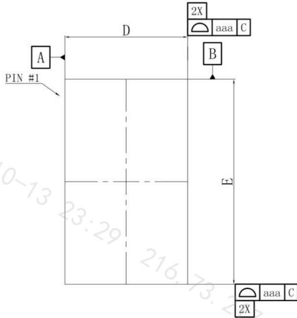
顶视图
