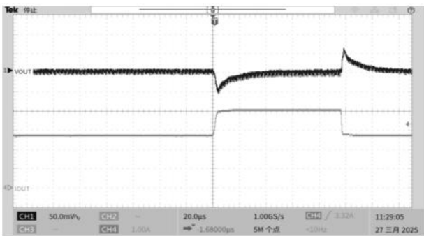
图 10. 2.5V 输出瞬态响应
