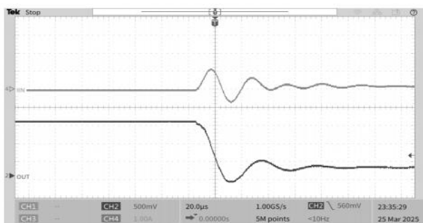
图 14. 空载短路
