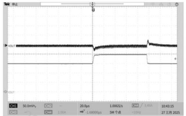
图 7. 1.2V 输出瞬态响应
