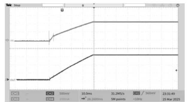
图 13. 3A 负载启动
