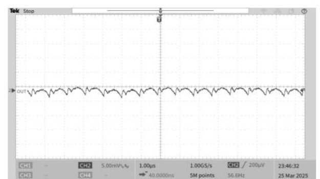
图 17. 输出纹波
