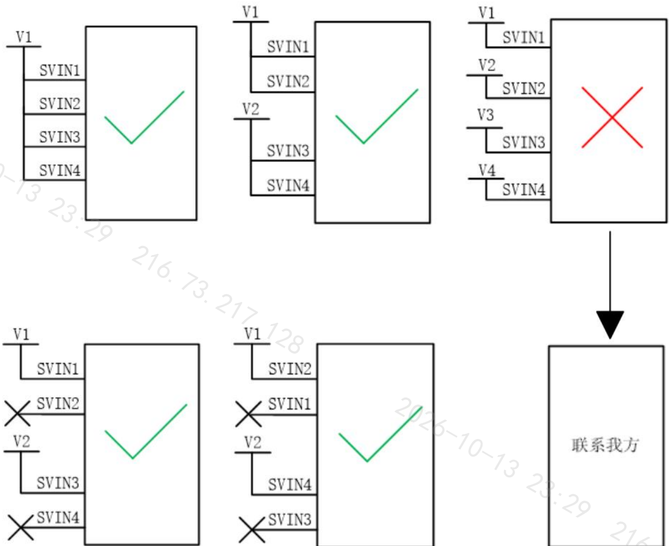
图 25. SVIN设计指示图
