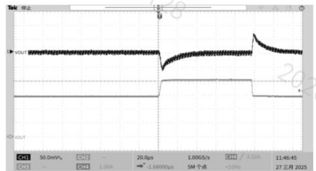
图 11. 3.3V 输出瞬态响应
