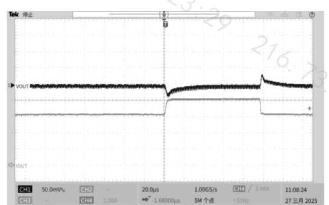
图 9. 1.8V 输出瞬态响应
