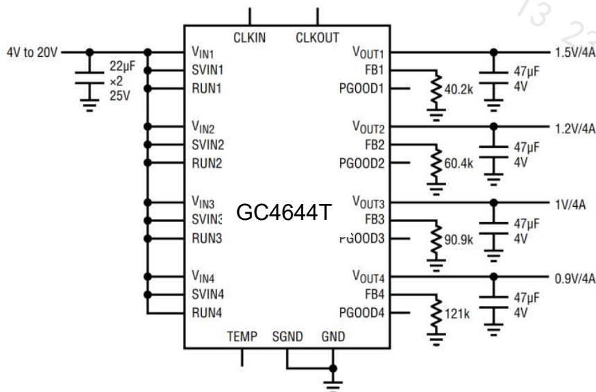
图 1. 典型应用框图
