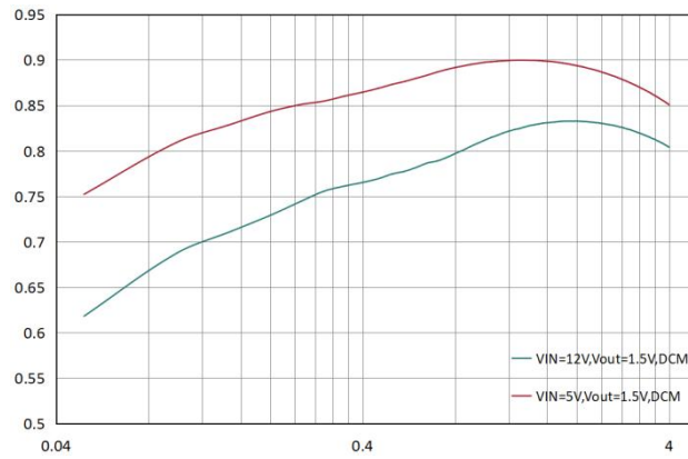
图 2. DCM 模式下效率曲线
