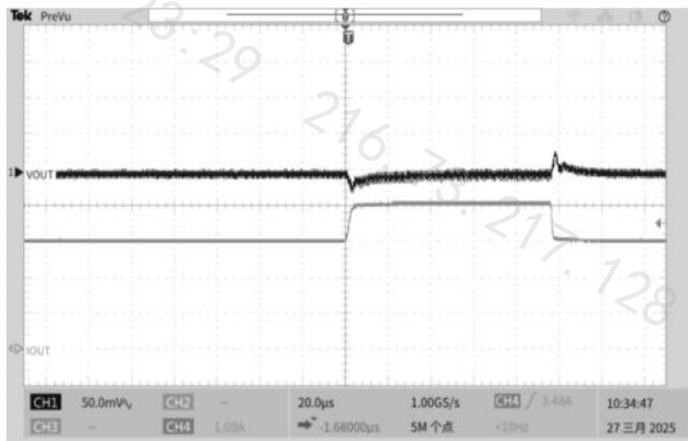
图 6. 1.0V 输出瞬态响应
