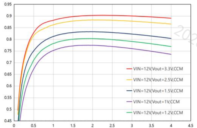
图 5. V_{IN}=12V , 效率曲线
