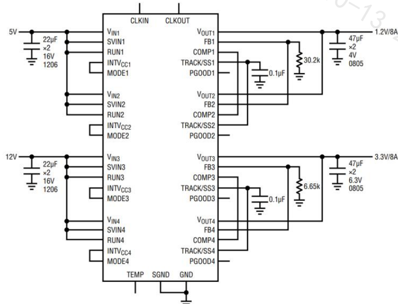
图 23. 12V 和 5V 两个独立的输入轨, 8A 输出 1.2V 和 8A 输出 3.3V
