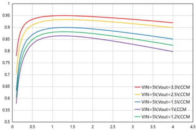
图 4. V_{IN}=5V , 效率曲线
