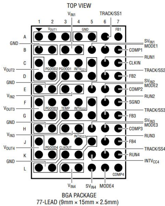
图 4. GC4644T 封装脚位图
