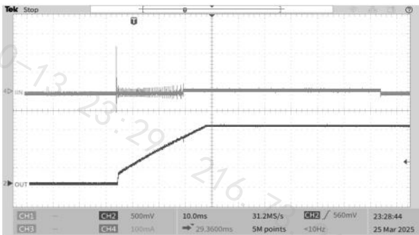
图 12. 空载启动
