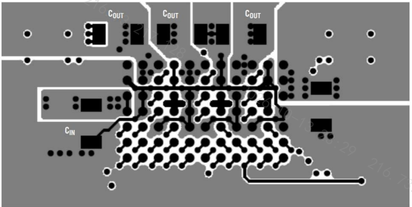
图 24. 推荐 PCB 布局
