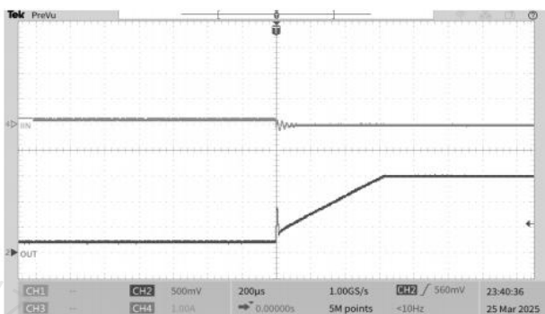
图 16. 3A 负载短路
