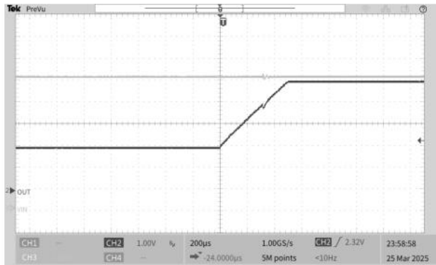
图 18. 启动预偏置输出
