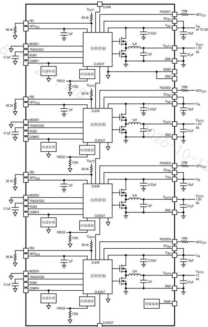
图 3. 功能框图
