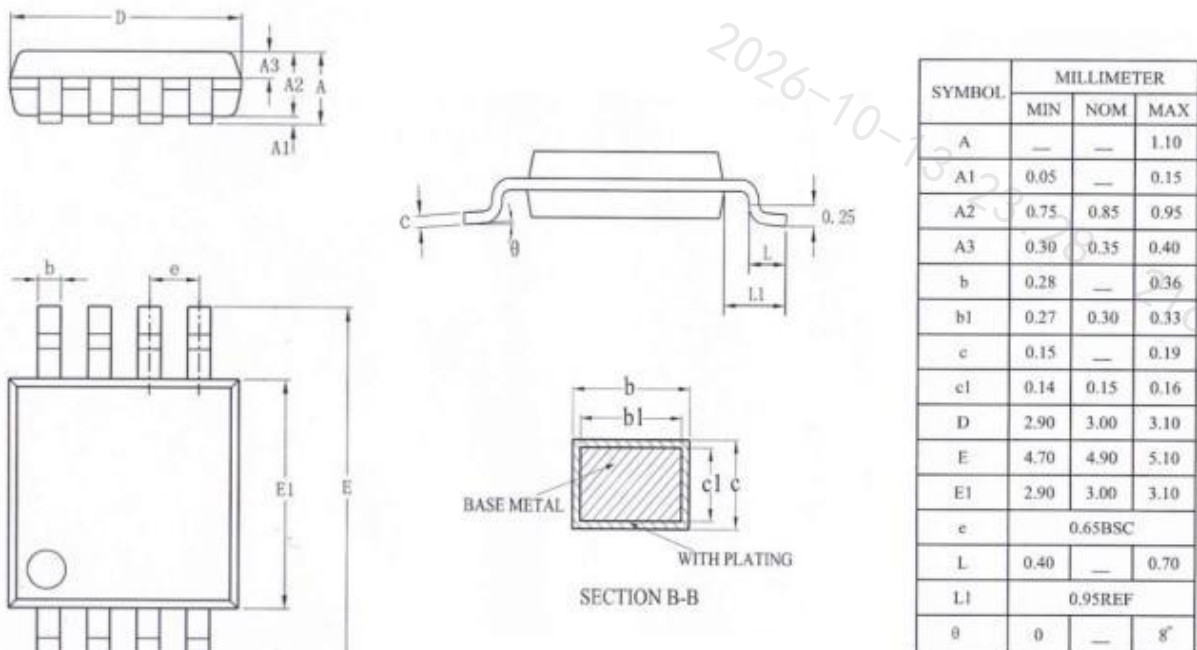
图 8 SOP8 封装尺寸
