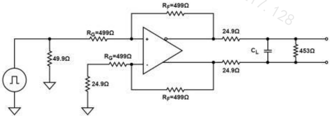
图 5 电容负载驱动测试电路
