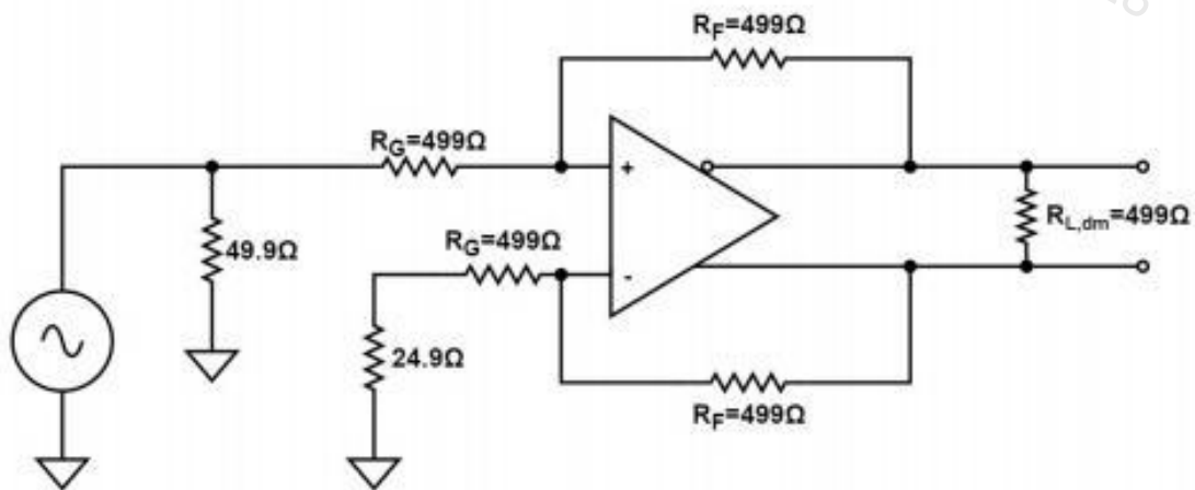
图 4 基本测试电路
