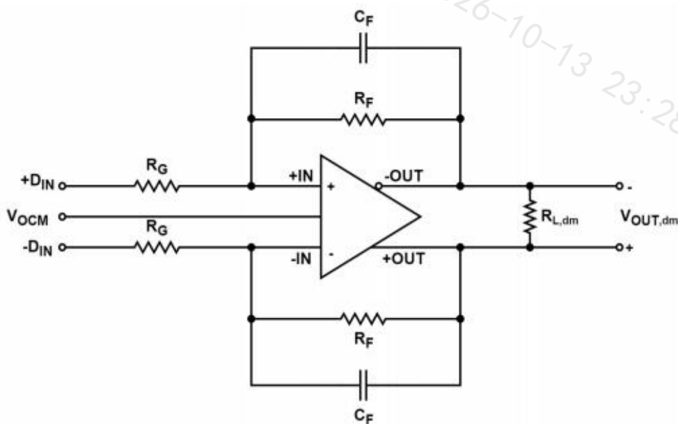
图 7 电路定义
