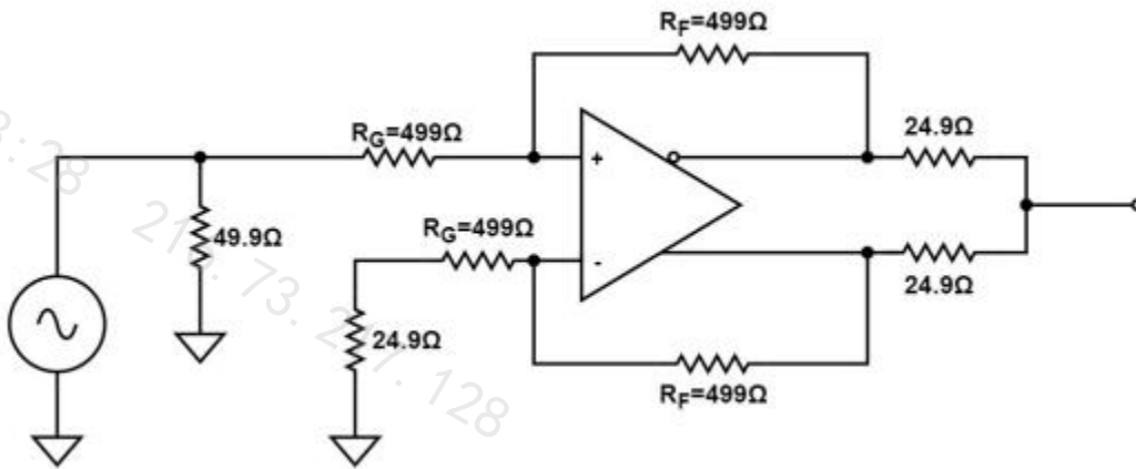
图 6 输出平衡测试电路
