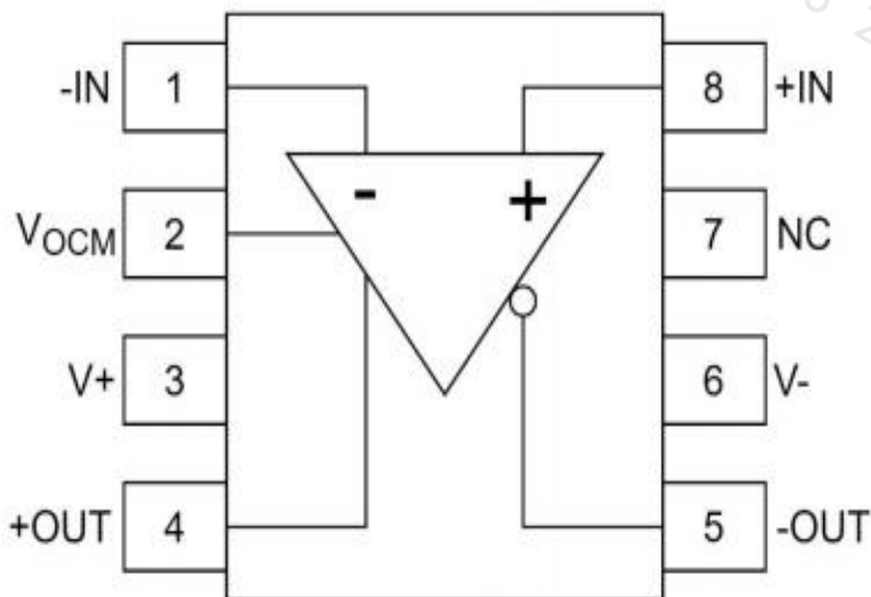
图 2 管脚配置
