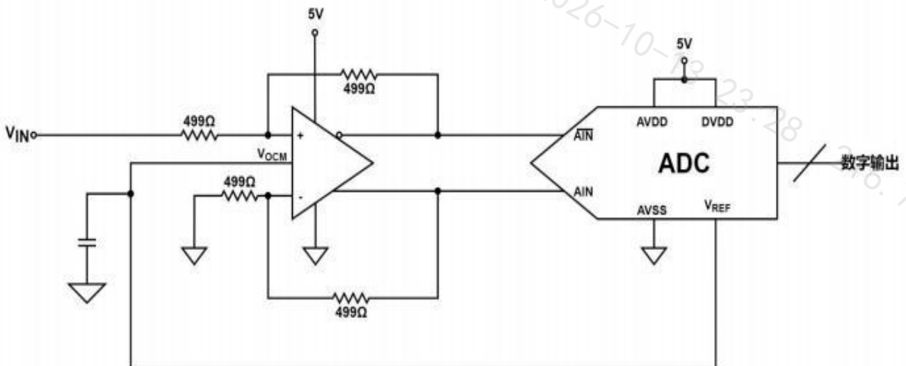
图 1 典型应用电路图
