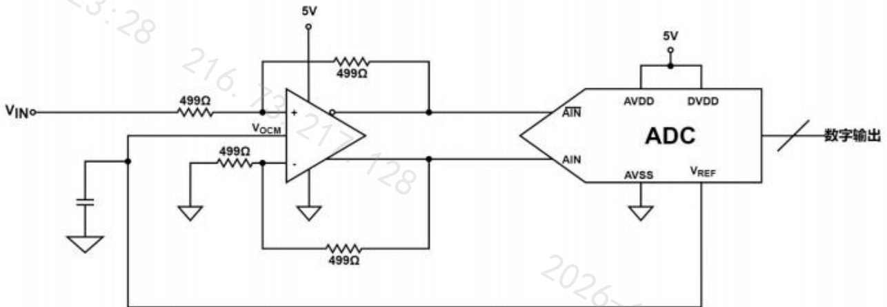
图 3 典型应用电路
