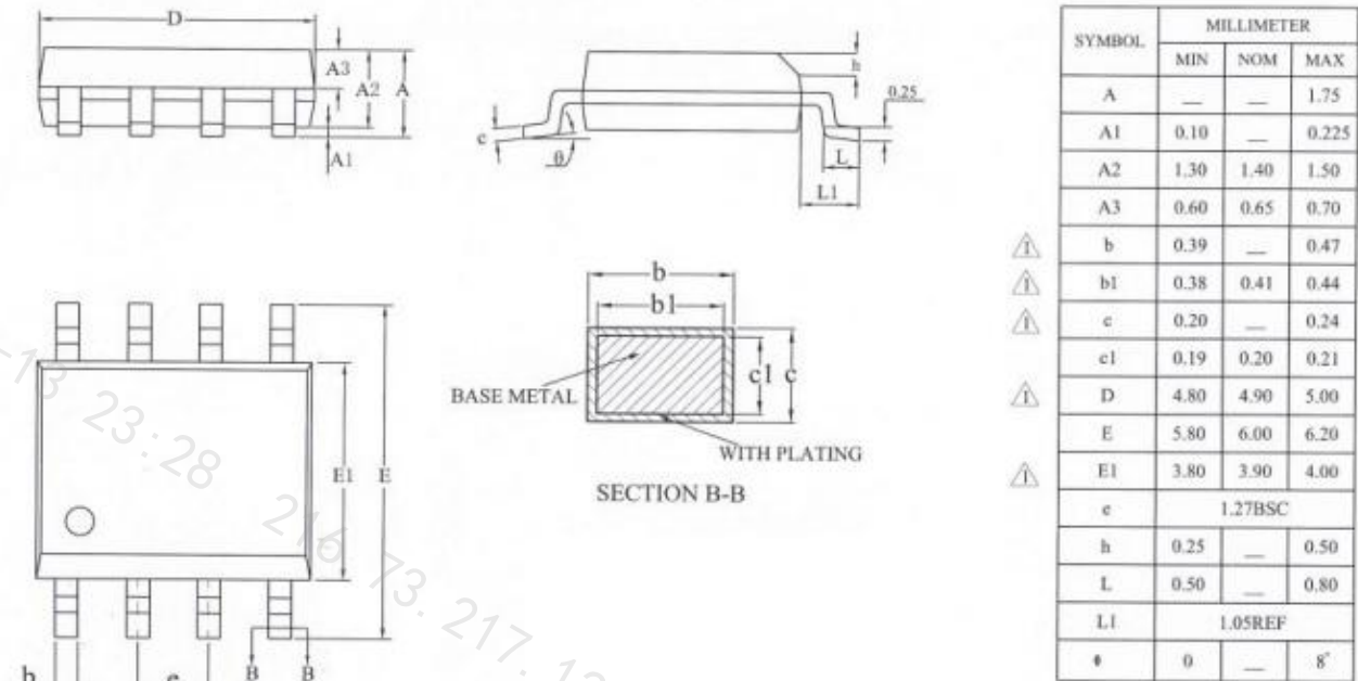
图 8 SOP8 封装尺寸
