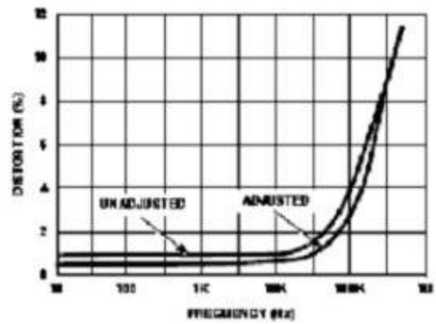
图 20 正弦波失调和频率
