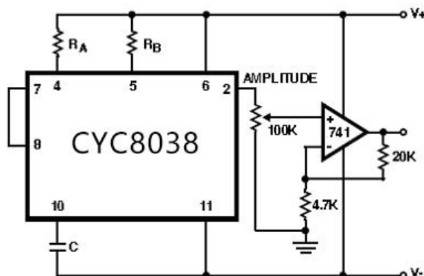
图 6 正弦波输出缓冲放大器
