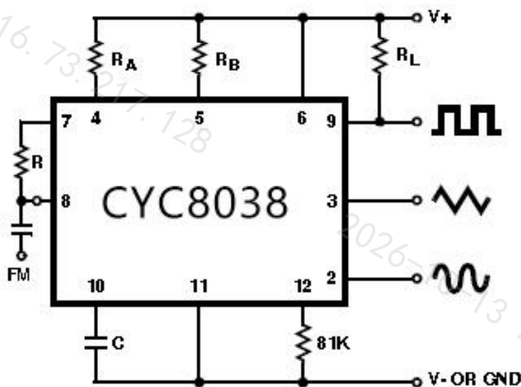
图 5 频率调制连接框图
