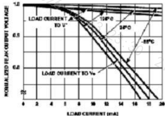
图 16 三角波输出电压和负载电流
