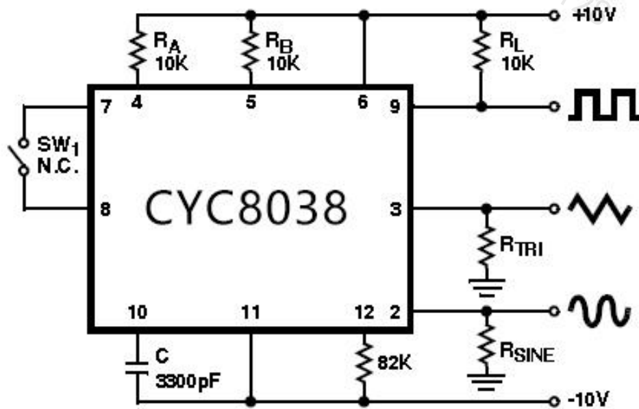
图 1 测试电路
