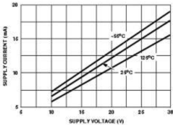
图 11 电源电流和电源电压
