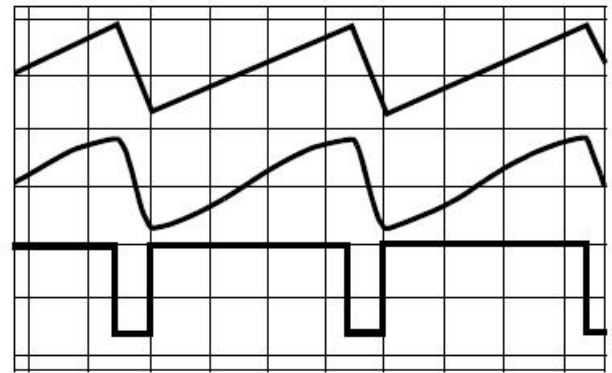
2B 方波占空比-80%
