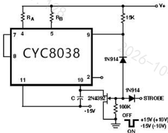
图 7 调制选通发生器
