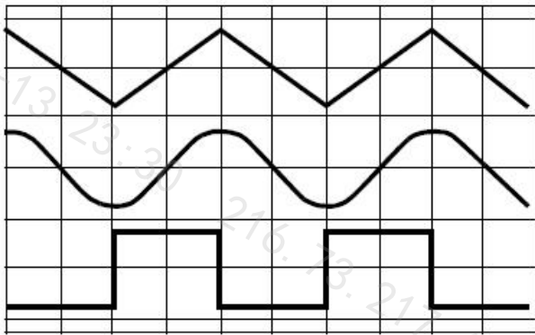
2A 方波占空比-50%
