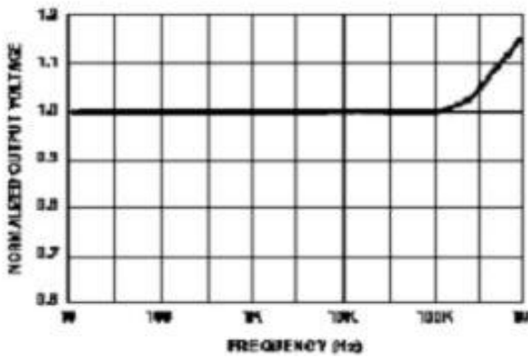
图 17 三角波输出电压和频率
