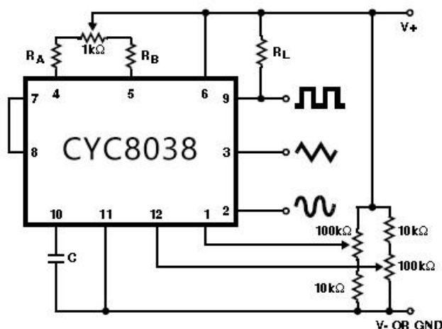
图 4 最小正弦波失真连接框图
