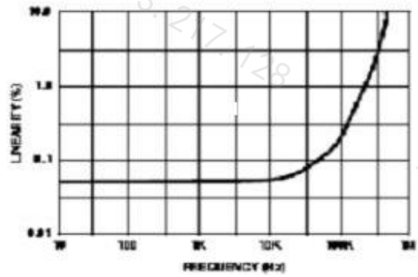
图 18 三角波线性度和频率
