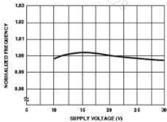
图 12 频率和电源电压
