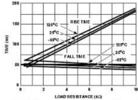
图 14 方波输出端上升/下降沿时间和负载电阻
